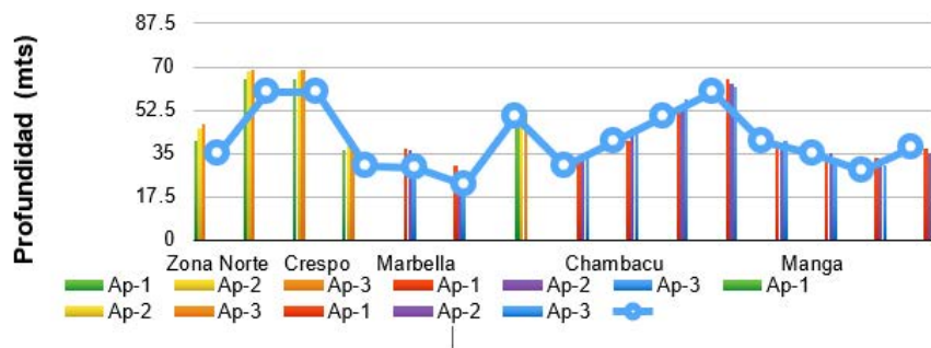
Figura 10. Nivel de Agua Freática según zona de Estudio. Profundidad de agua freática.
