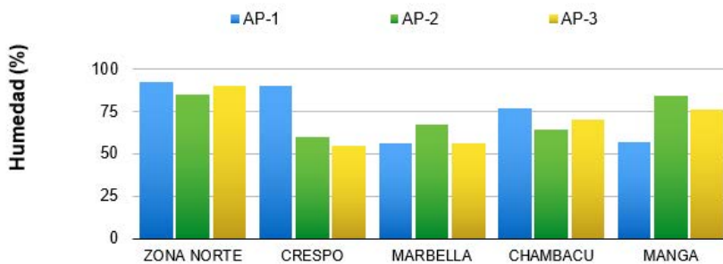
Figura 11. Contenido de Humedad muestras recuperadas a 1,0 m de profundidad.
